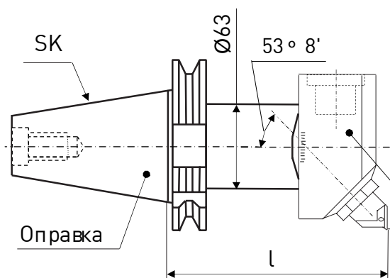
Угловая установка микробора
