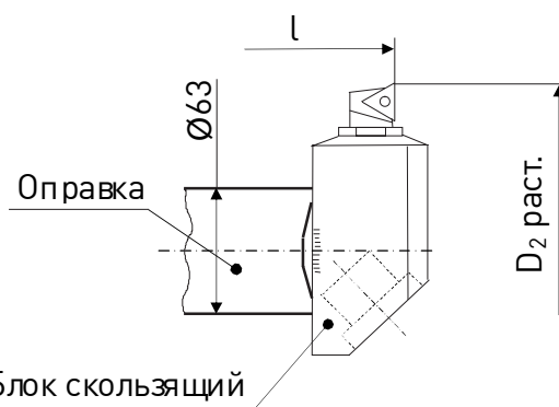
Радиальная установка микробора
